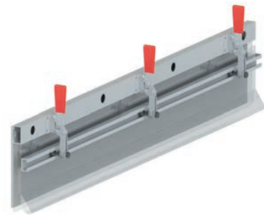
Staubdichtung passt sich der Gurtmuldung an
